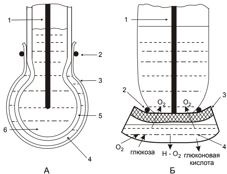
Рис. 3.5. Ферментные электроды (по Н. Н. Угаровой, 1987).
