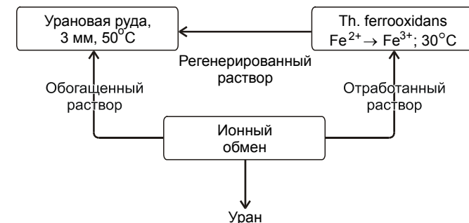
Рис. 5.5. Схема выщелачивания урановой руды (по J. Johnson, 1985).
