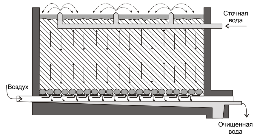
Рис. 7.1. Схема биофильтра (по М. С. Мосичеву и др., 1982).
