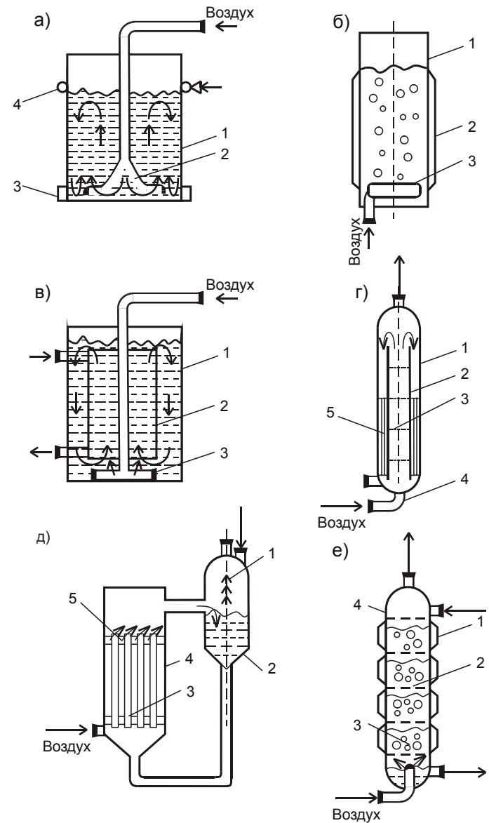
Рис. 1.6. Ферментеры с подводом энергии газовой фазой (группа ФГ) (Виестур и др., 1986). а) барботажный: 1 – корпус, 2 – воздухораспределитель, 3 – карман, 4 коллектор, б) барботажный колонный: 1 – корпус, 2 – рубашка, 3 – воздухораспределитель, в) барботажно-эрлифтный: 1 – корпус, 2 – диффузор-теплообменник, 3 – воздухораспределитель; г) газлифтный: 1 – корпус, 2 – диффузор, 3 – диспергатор, 4 – воздухораспределитель, 5 – теплообменник, д) трубчатый: 1 – пеногаситель, 2 – емкость, 3 – диспергатор, 4 – корпус, 5 – распределительная перегородка, е) с плавающей насадкой: 1 – рубашка, 2 – тарелка, 3 – насадка, 4 – корпус.
