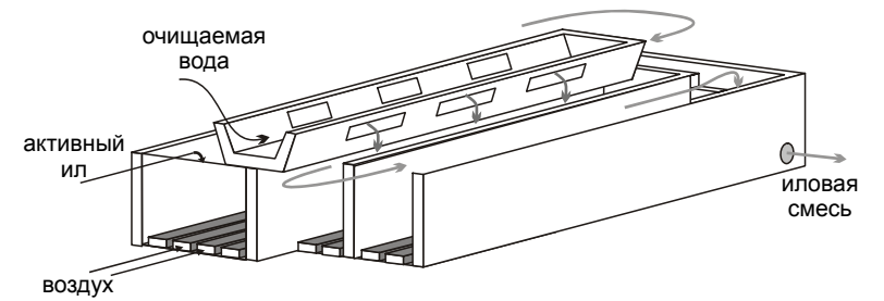
Рис. 7.3. Схемы аэротенков.
