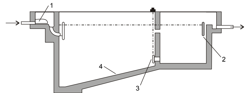
Рис. 7.4. Двухкамерный септиктенк (по К. Форстеру, 1990). 1 – регулятор, 2 – отрагатель, 3 – напорный трубопровод, 4 – уклон 1:4.
