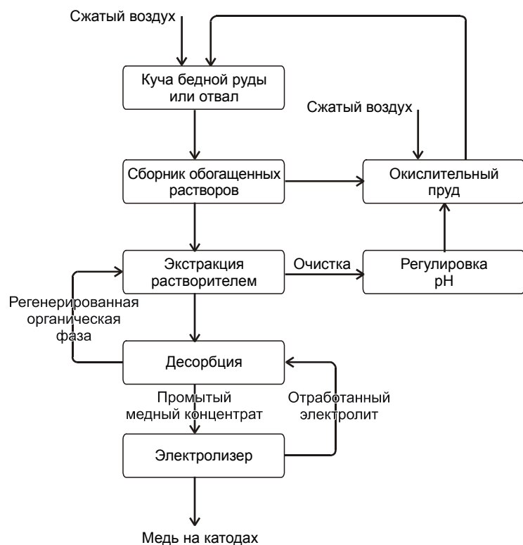
Рис.5.4. Схема бактериального выщелачивания меди из куч или отвалов руды (по Ф. Д. Пули, 1990).
