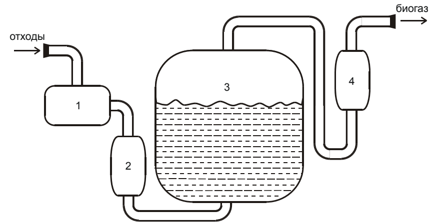
Рис. 1.5. Схема метановой установки. 1 – дозирующее устройство, 2 – теплообменник, 3 – метанотенк; 4 – газгольдер.
