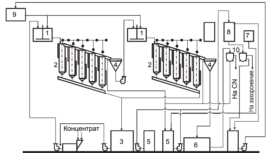
Рис. 5.6. Схема установки чанового выщелачивания металлов (по Г. И. Каравайко, 1984). 1 – контактный чан, 2 – пачук, 3 – чан для сбора оборотных растворов, 4 – обезвоживающий конус, 5 – чан для сбора остатка после выщелачивания, 6 – отстойник конечного продукта, 7 – подача известкового молока, 8 – чан-отстойник, 9 – чан для сбора оборотных растворов, 10 – нутч-фильтр.
