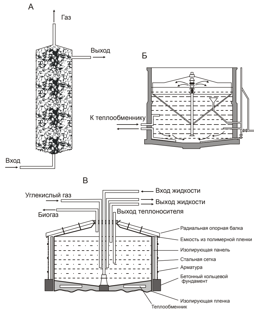
Рис. 7.5. Типы установок для очистки сточных вод пищевой промышленности. А – анаэробный биофильтр, Б – установка с винтовым насосом для перемешивания, В – высокоскоростной реактор Коулзера (по Дж. Бесту и др., 1988).
